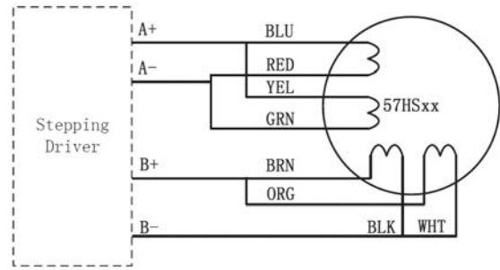
(d) 57HSxx parallel connection (8 leads)
